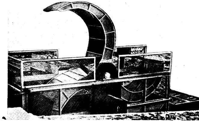
Рисунок 5.24 - Рыбоперегрузатель передвижной УППР
